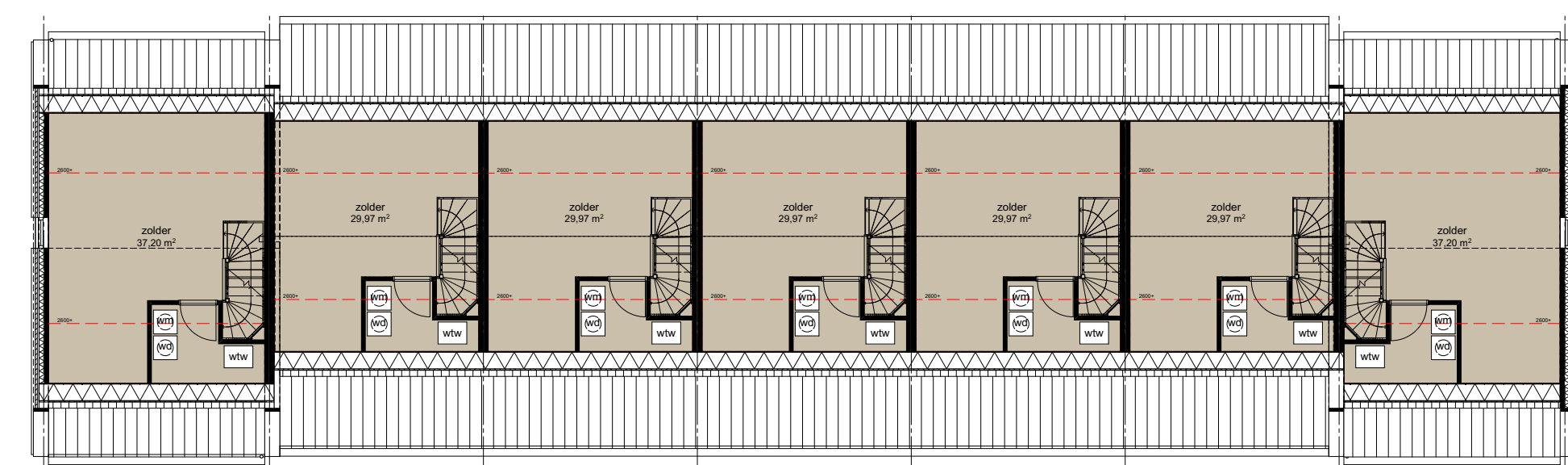
Tweede verdieping
